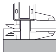
Elmozdulásmérés
