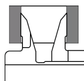
Vnitřní měření
