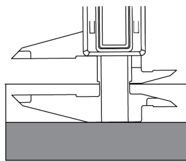
Krokové měření
